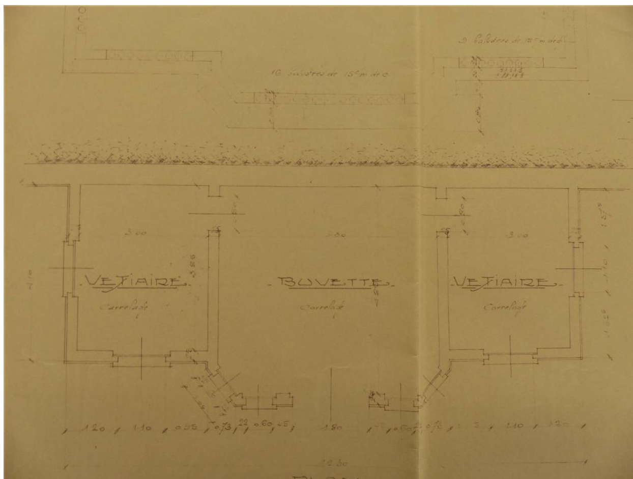
Ville de Roye. Société de Longue paume de Roye. Reconstruction du châlet et de la tribune du jury. Châlet : plan au sol. A. Coël architecte, 1927 (AD Somme ; 99O 3297).
