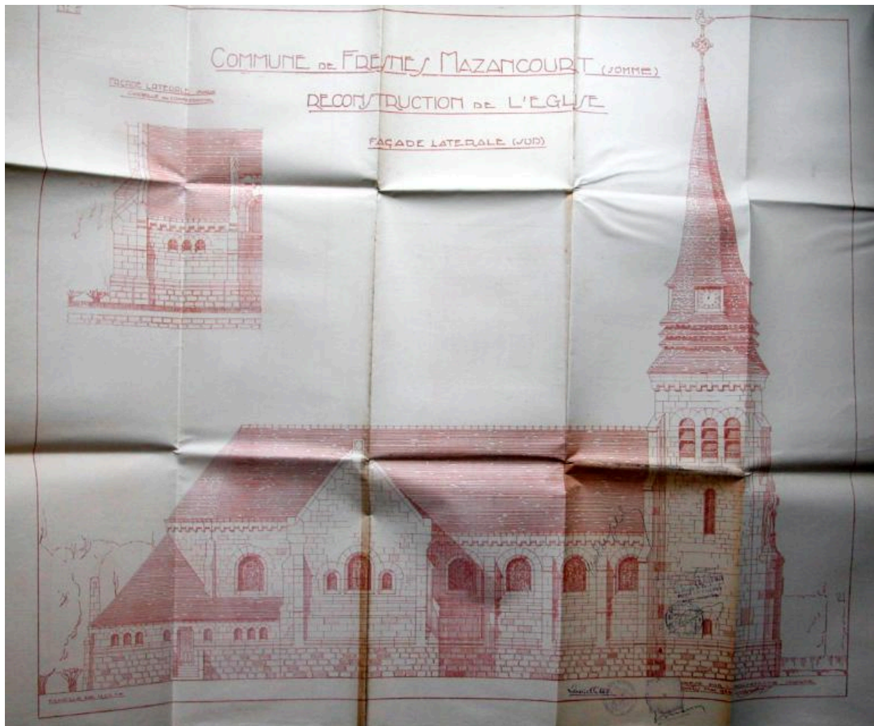
Elévation de la façade latérale sud, Louis Duthoit (architecte), avril 1928 (AD Somme ; 99 O 1846).
