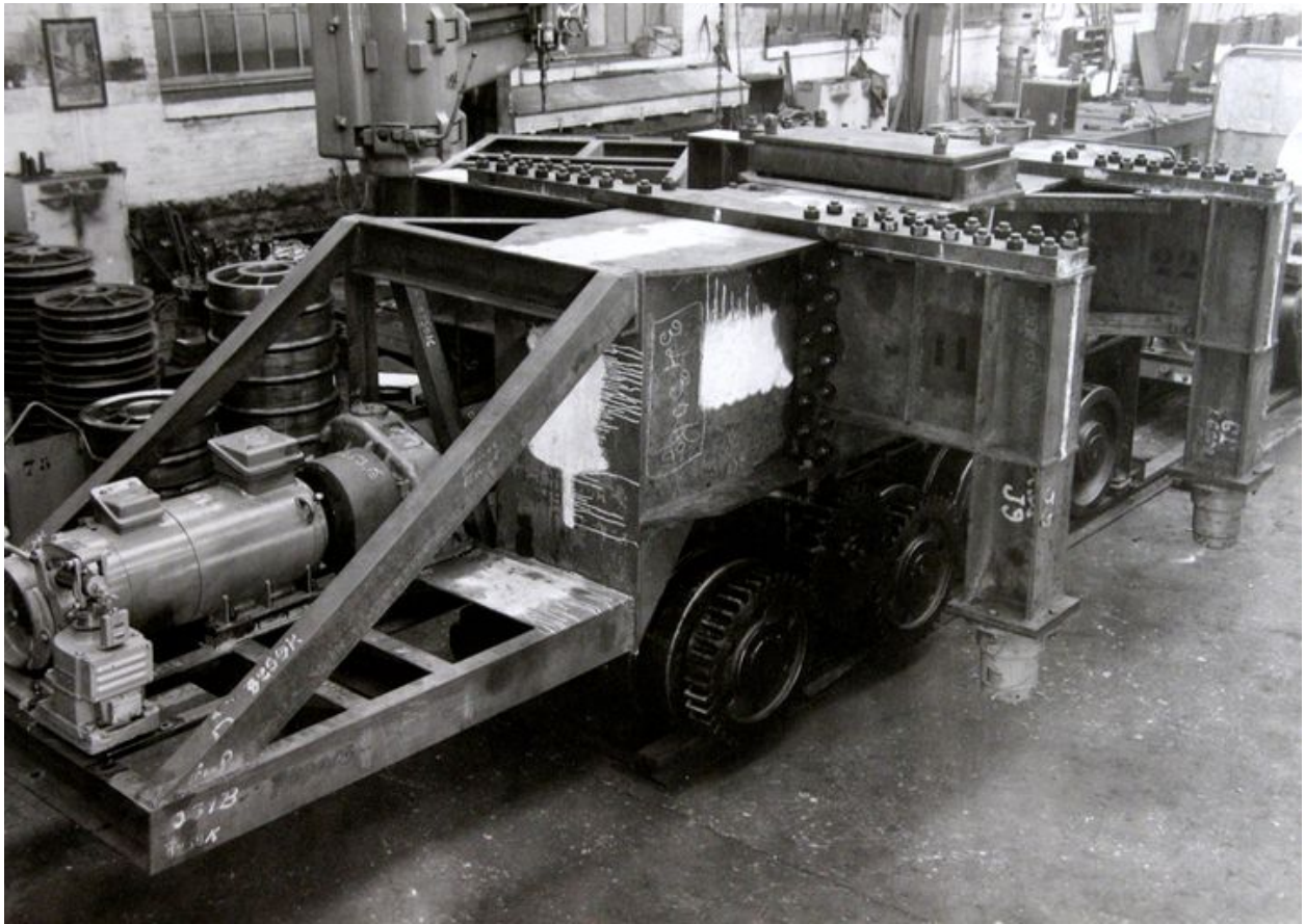
Ensemble d'un boggie construit pour Usinor à Dunkerque, 1962 (AP).
