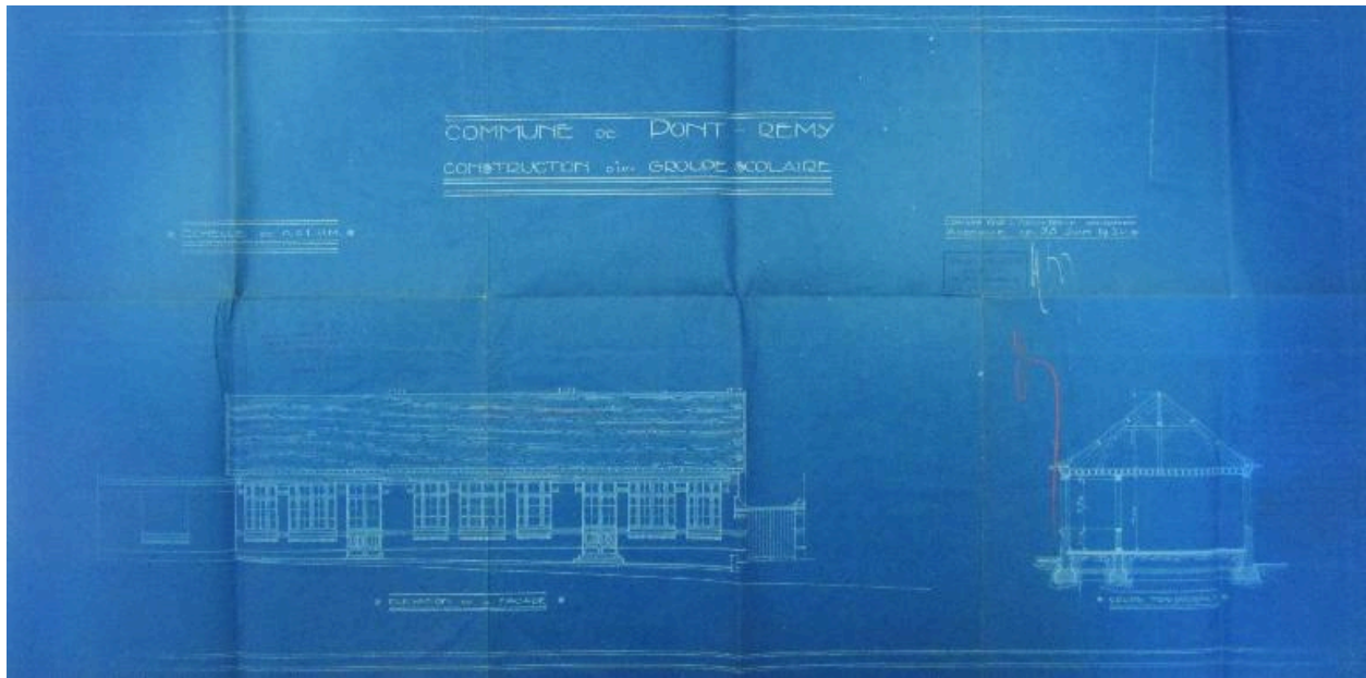
Elevation de la façade et coupe transversale du groupe scolaire, Marcel Digeon (architecte), 28 juin 1930 (AD Somme ; 99 O 3079).
