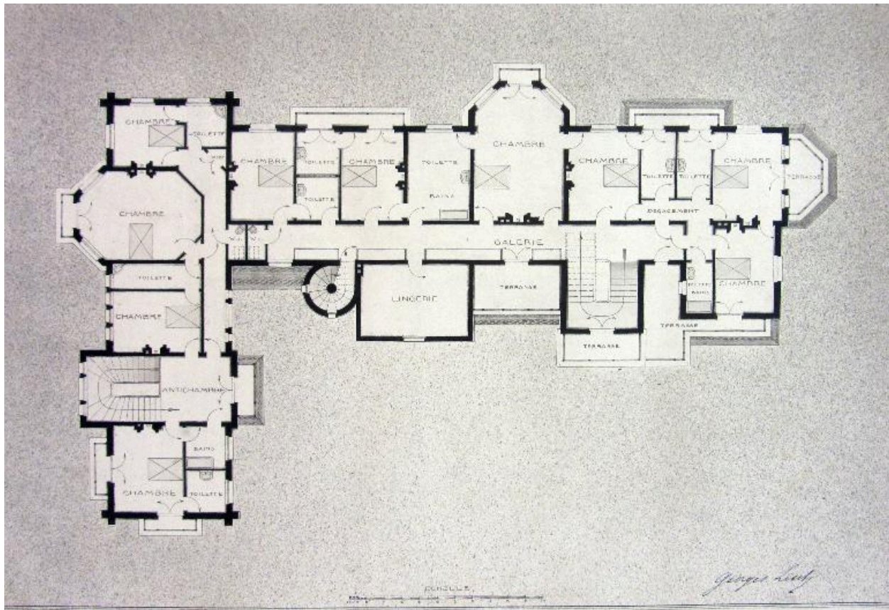
Plan du premier étage de la maison de directeur, Georges Lisch, architecte (AD Somme ; 49 Fi 8)
