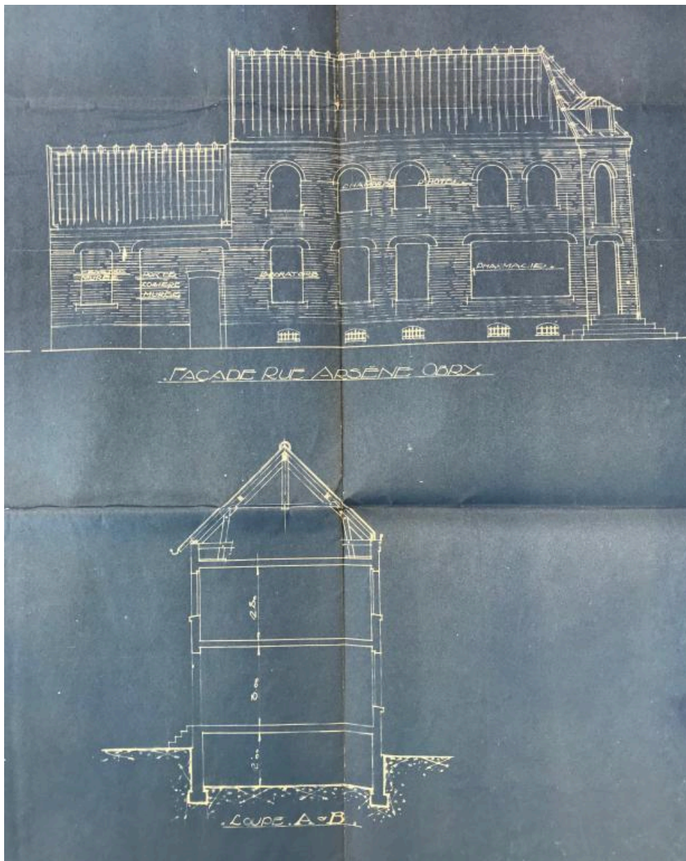
Société coopérative de l'Union à Villers-Bretonneux. Façade rue Arsène-Obry et coupe, 1922 (AD Somme ; 10R 1250).
