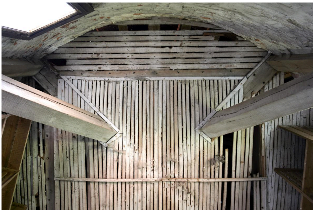
Niveau supérieur. Tour de guet. Détail du plafond en lattis de bois peint.
