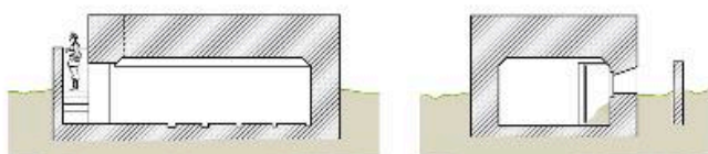
COUPE LONGITUDINALE B-B
