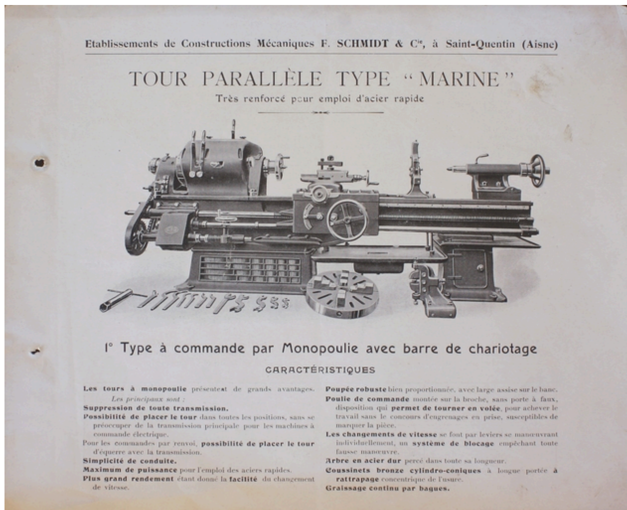
Tour parallèle type Marine construit avant 1914 par F. Schmidt & Cie (AD Aisne).
