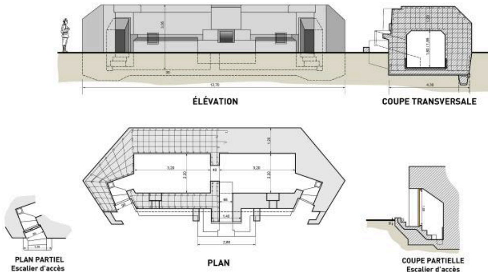
Abri avec position pour mitrailleuse 2 ème ligne secteur 7
