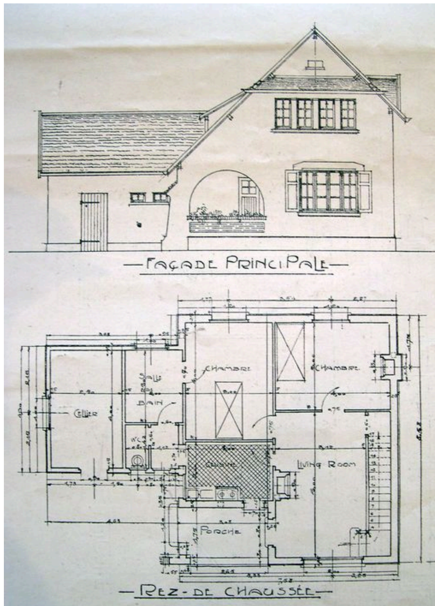
Type de maison à 1 logement de 6 pièces (pl. 25). Façade principale et plan du rez-de-chaussée. La construction Moderne, n° 4, 24 octobre 1926
