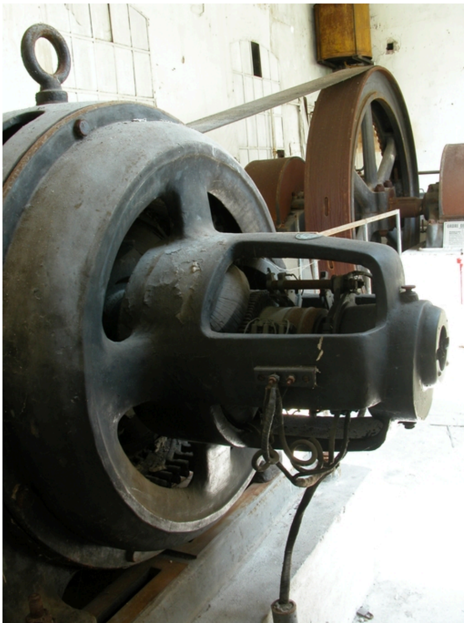
Générateur Schneider & Cie : détail de la dynamo.
