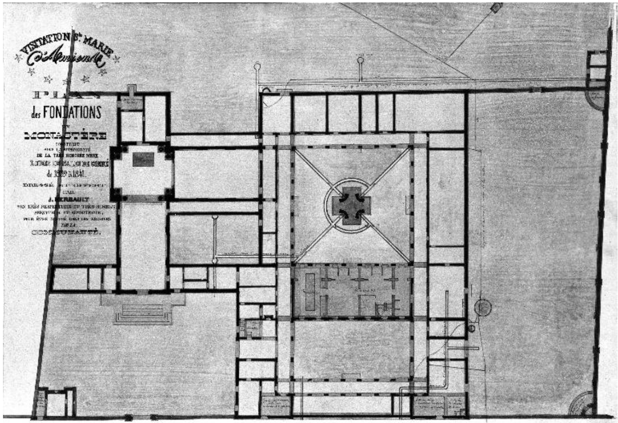
Visitation Sainte-Marie. Plan des fondations, dessin par J. Herbault, 1839-1841 (coll. part.).
