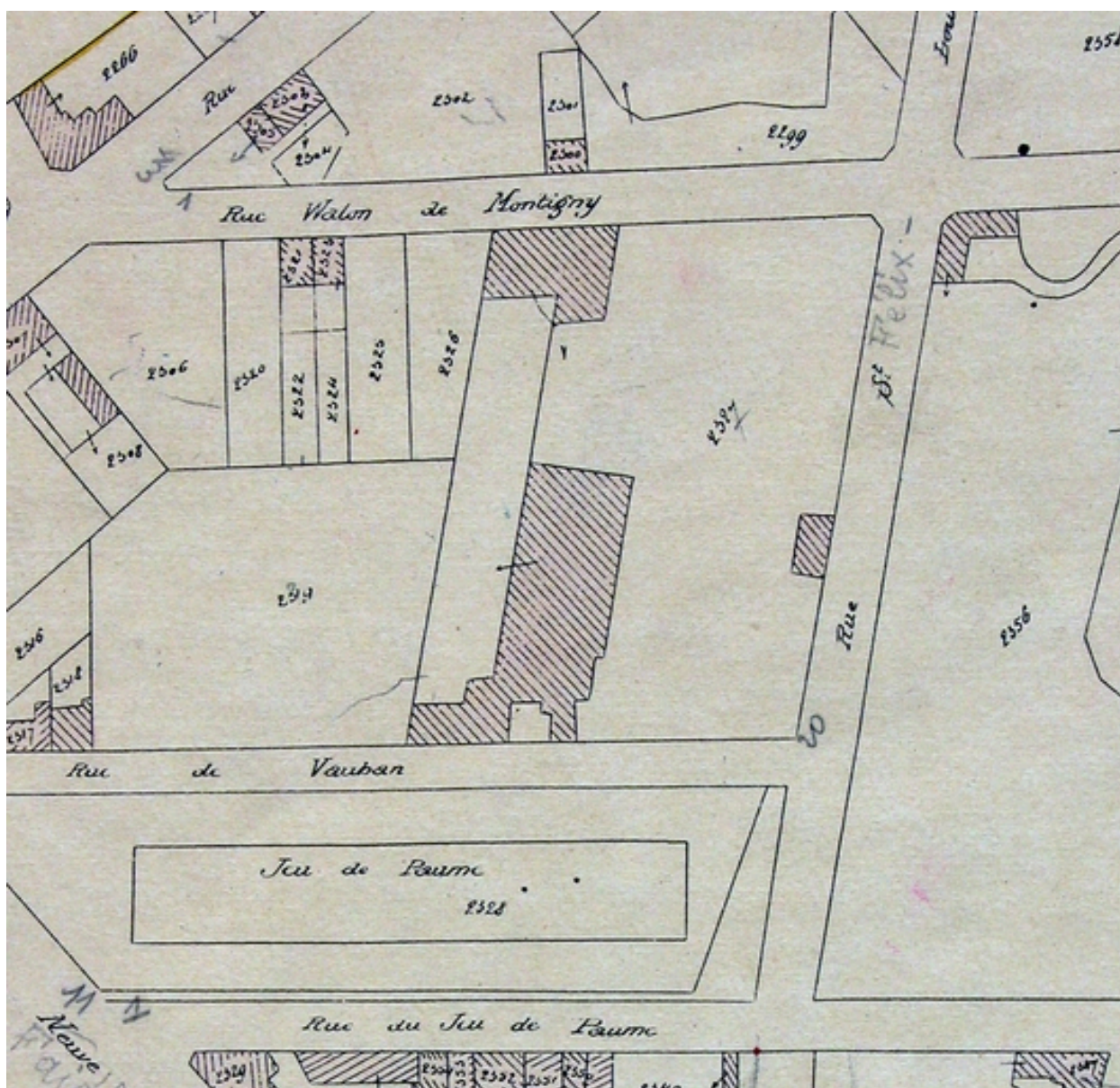
Plan masse de la Fabrique des Anglais avant 1831. Cadastre ancien, supplément à la section D de la ville. 3e feuille - n°1861 à 2391, parcelle n°2327 (AC Saint-Quentin).
