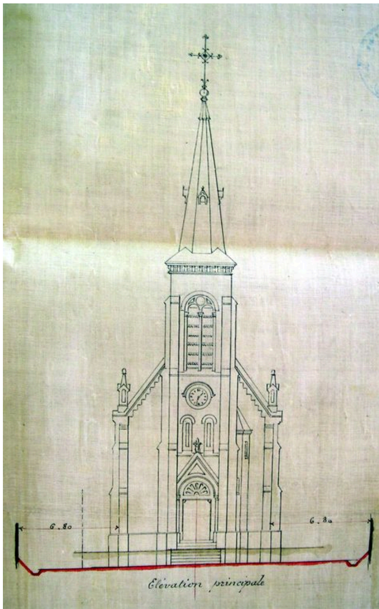
Élévation principale, Henry Antoine, juillet 1887 (AD Somme ; 5 V 54).
