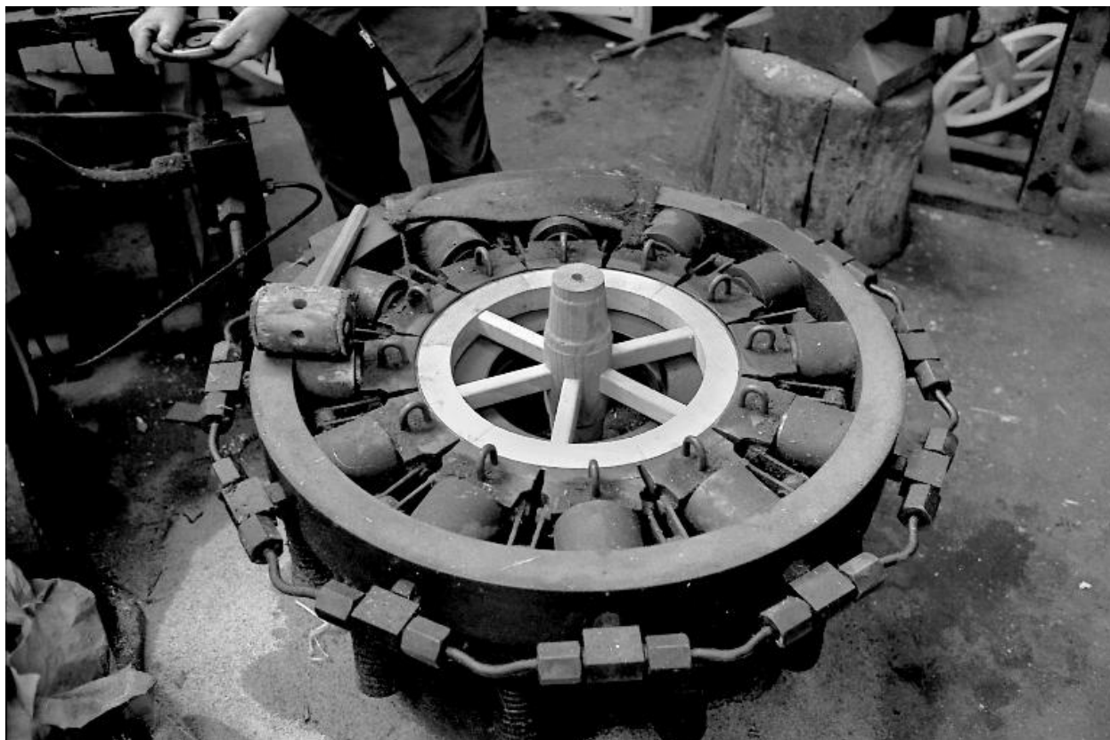
Atelier de fabrication, vue intérieure en 1990. Machine à lever les roues.
