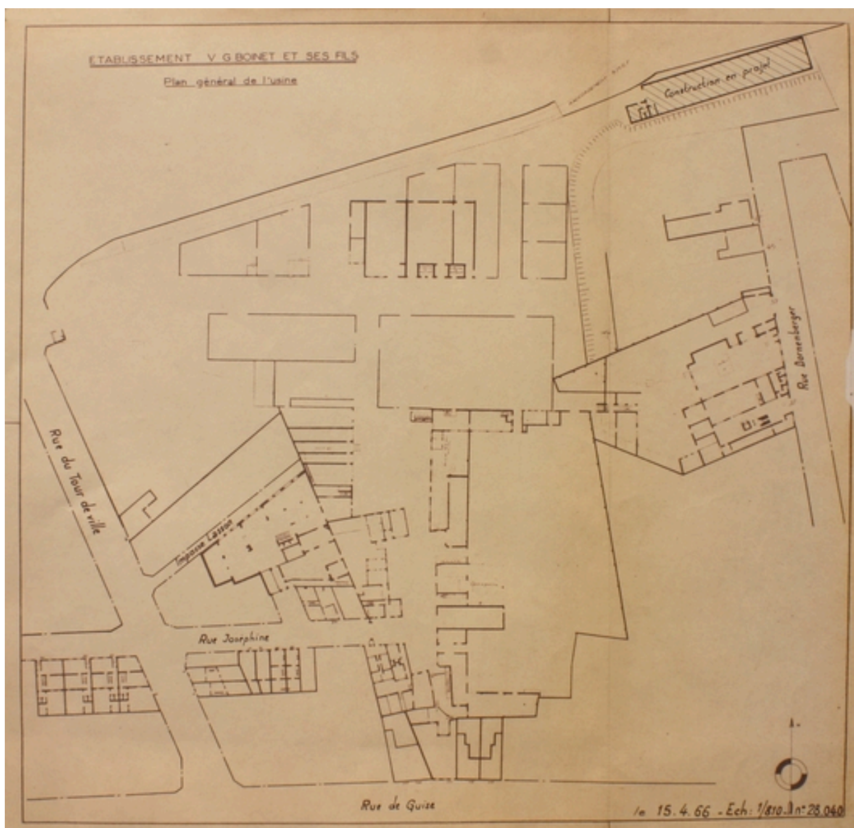
Plan masse de l'usine en 1966 (AC Saint-Quentin).
