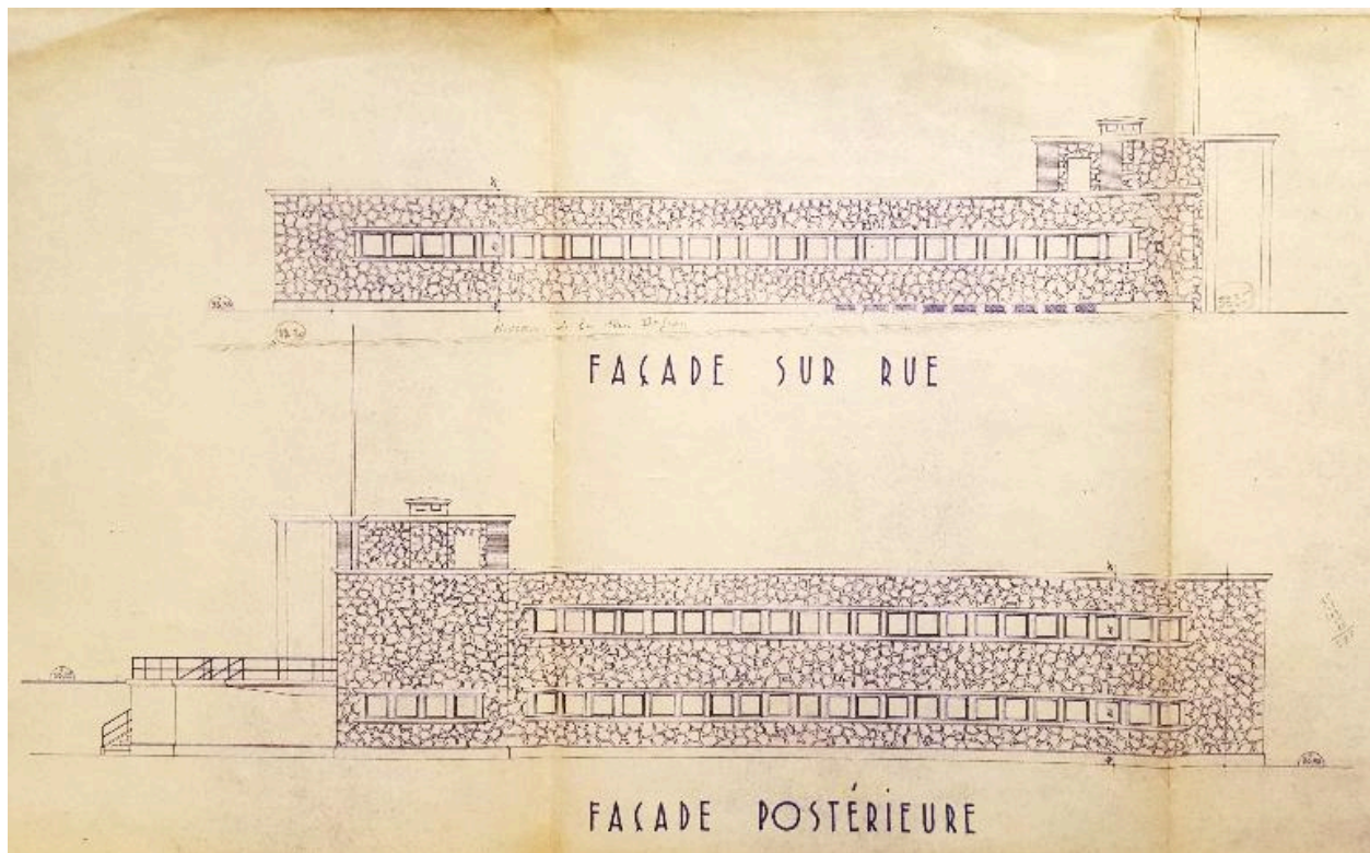
Avant-projet, plan de la façade sur rue et de la façade postérieure, 4 février 1947, A. et P. Dufau (IFA ; 066 1025/5).
