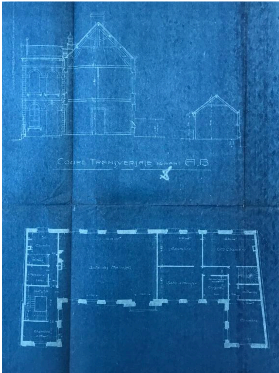
Villers-Bretonneux. Mairie. Plan du rez-de-chaussée, 1920 par A. Guilbert (AD Somme ; 10R 1250).
