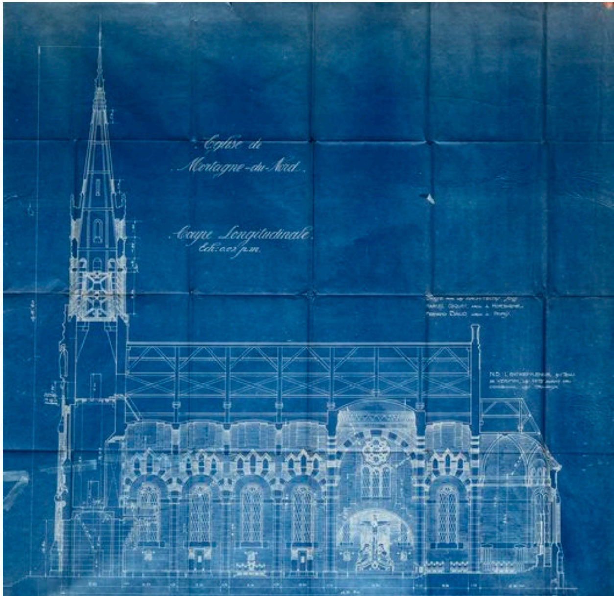
Coupe de l'église, Fernand Baud et Marcel Coquet architectes, 1924 (AD Nord, 20421/200).
