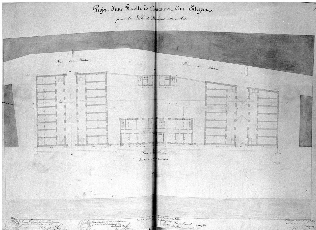
Douane, entrepôt public, plan du rez-de-chaussée, éch. 0,01 p.m. B.M. Boulogne-sur-Mer, ms 535 P. pl. 7.
