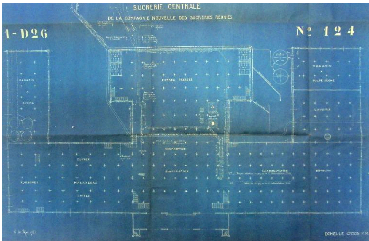
Plan détaillé de l'atelier principal de la sucrierie, 19 mai 1921 (AD Somme ; 5 M 623).
