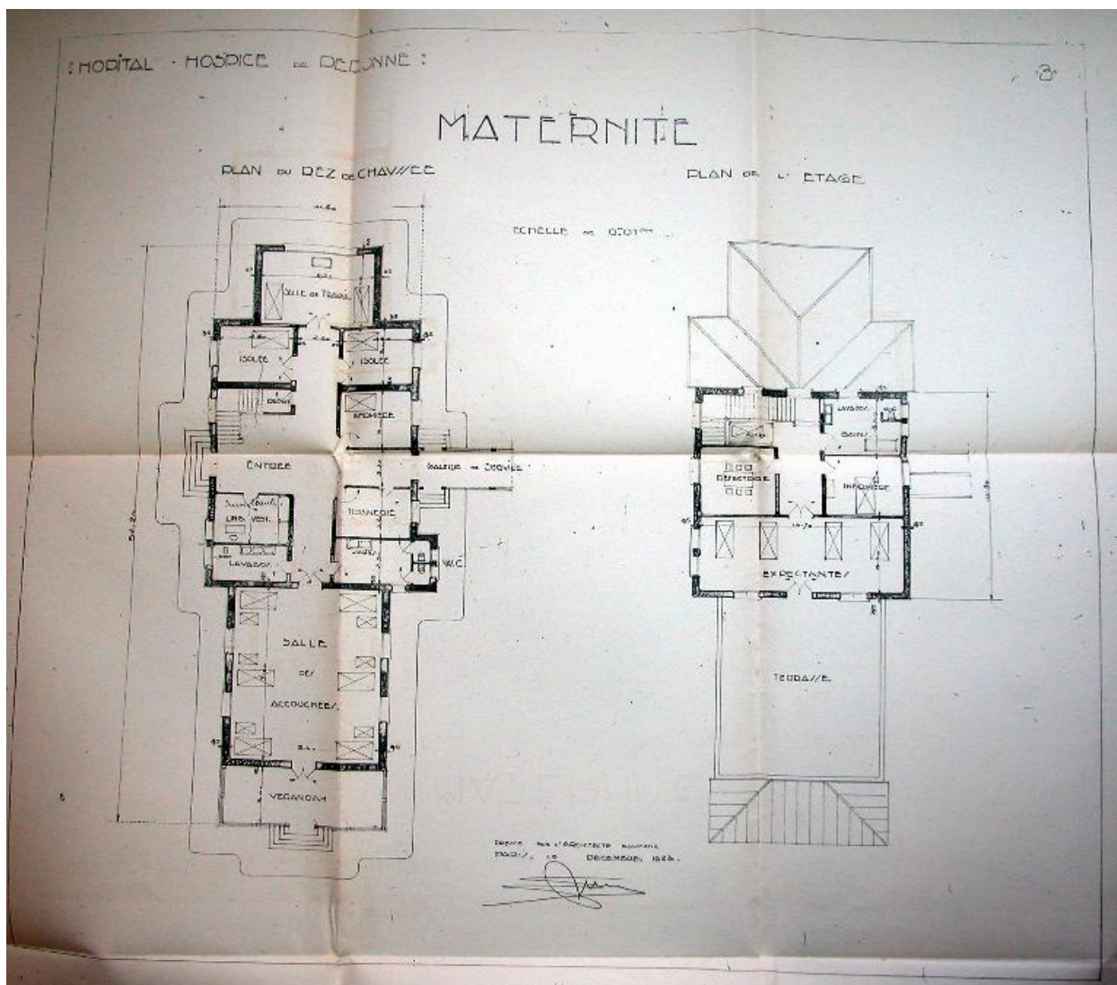
Projet de reconstruction de l'hôpital-hospice de Péronne, Pavillon de la maternité : plan du rez-de-chaussée et de l'étage, Jacquet Georges (architecte), décembre 1923 (AD Somme ; 10 R 1033).
