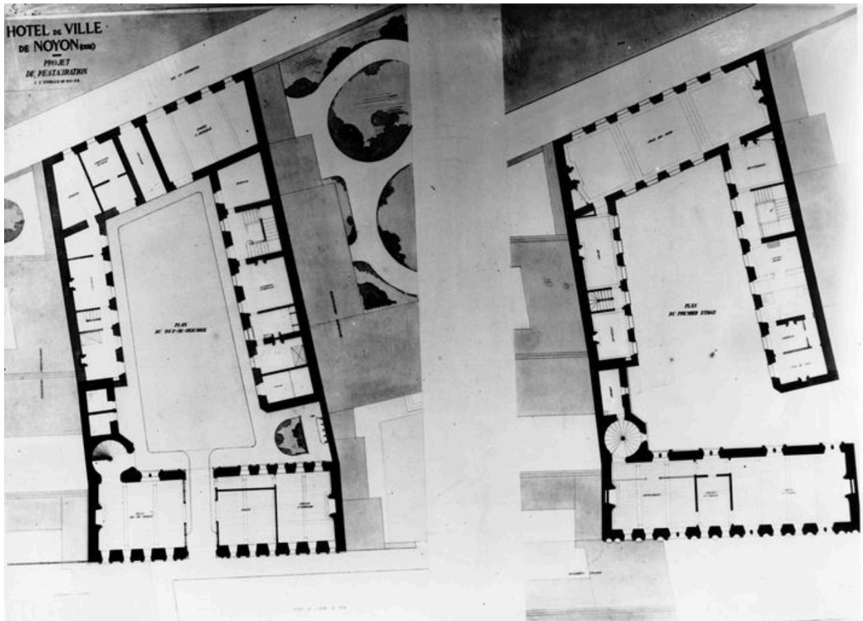
Projet de restauration. Plan du rez-de chaussée et du premier étage, par Seltersheim, 1882.
