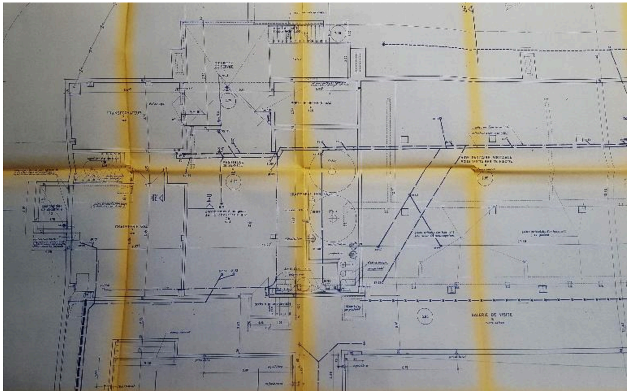
Plan du sous-sol : détail des locaux techniques de la piscine, Maurice Ego architecte, 1968 (AC Saint-Omer ; 3W40).
