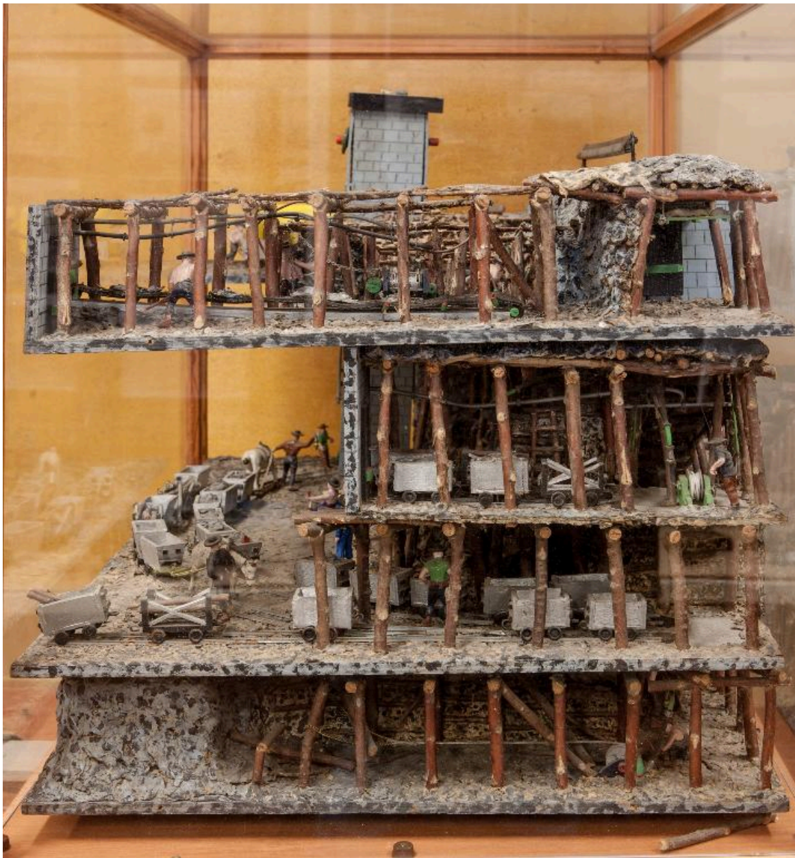
Vue latérale de la maquette présentant un chantier de boisage avant 1950 d'une galerie de mine réalisée par Jean Cathelain, habitant-paysagiste à Billy-Montigny. Maquette visible au musée de la Mine d'Oignies.
