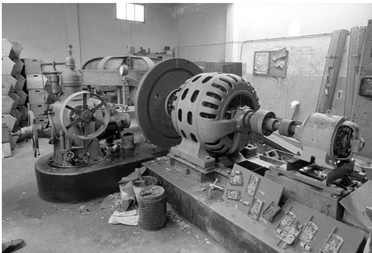
Bâtiment d'eau, vue intérieure : turbine hydraulique et alternateur.
