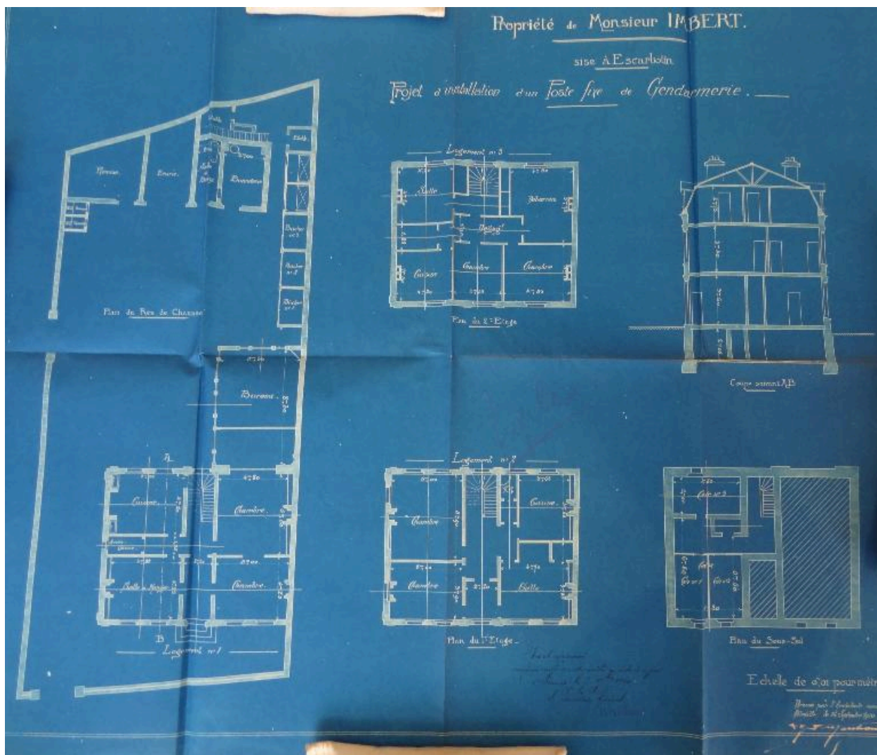
Plan de la demeure Imbert, par l'architecte A. Marchand, 1910 (AD Somme ; 990 1904).
