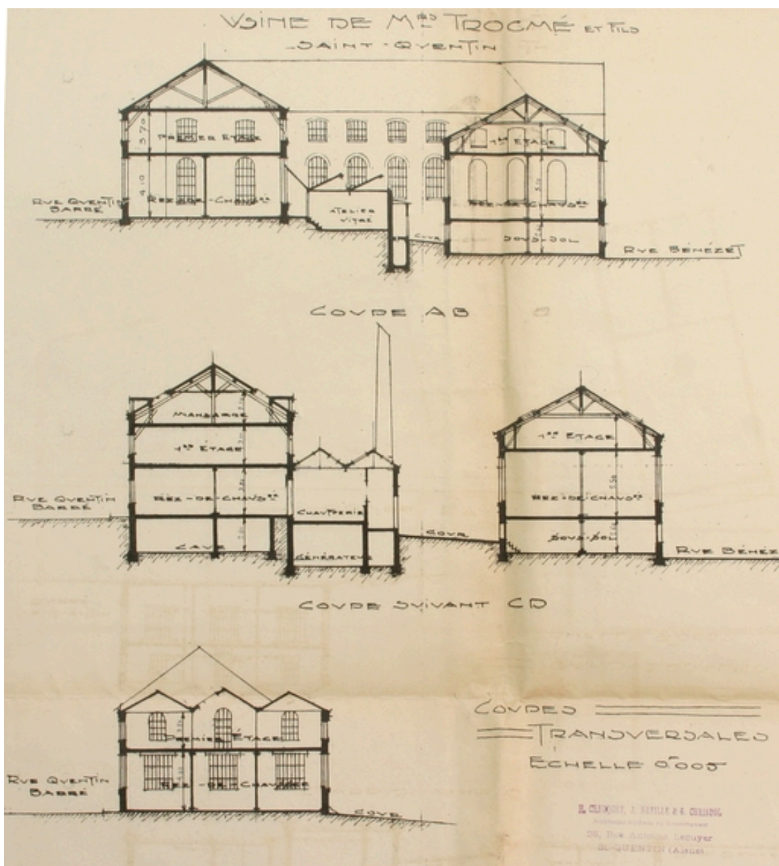
Coupes transversales de l'usine Trocmé à la veille de la Première Guerre mondiale, dressées après 1919 par Chauquet, Navile et Christol (AD Aisne).
