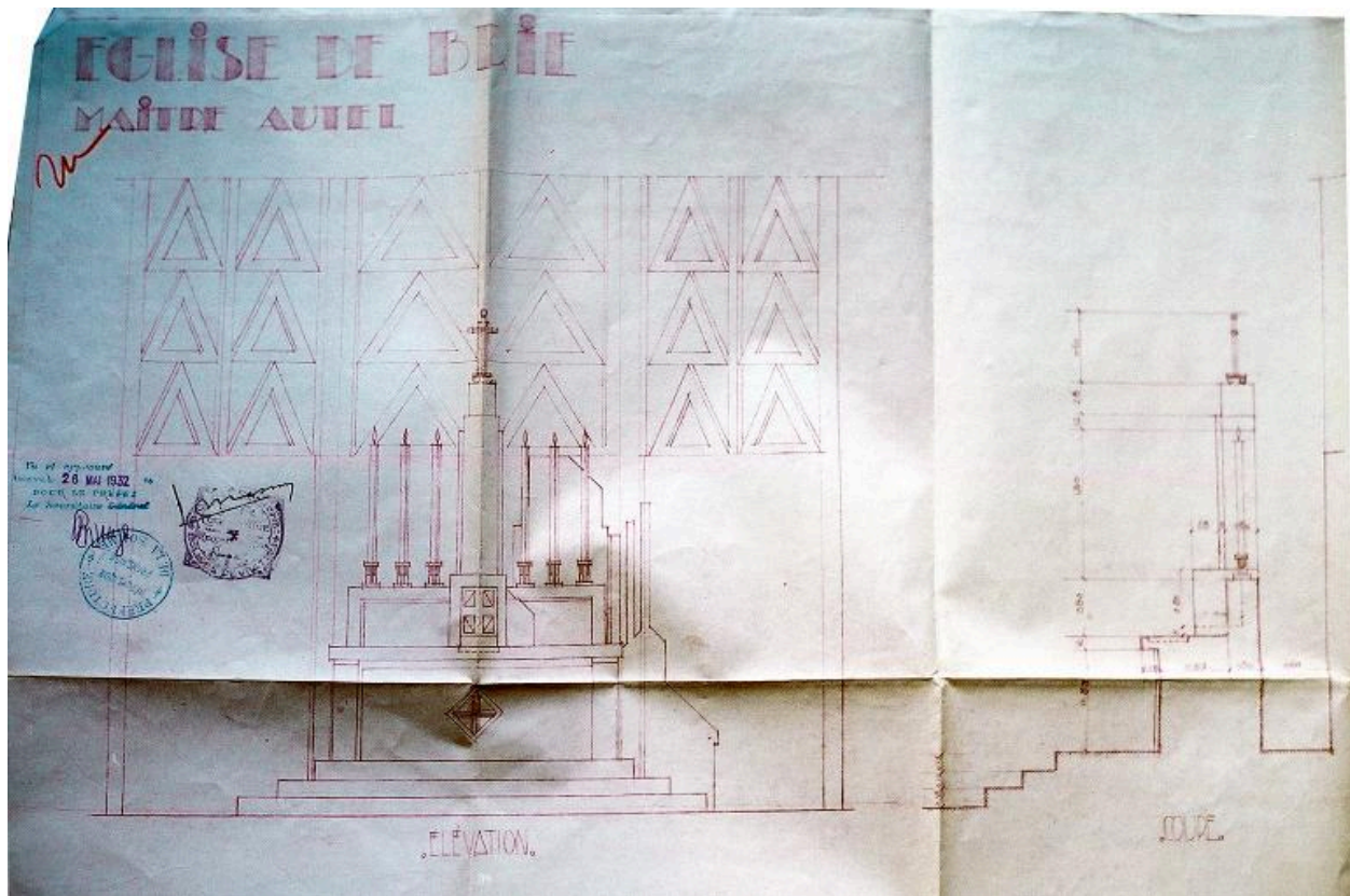
Coupe et élévation du maître-autel, Jacques Debat-Ponsan (architecte), 16 juillet 1931 (AD Somme ; 99 O 902).
