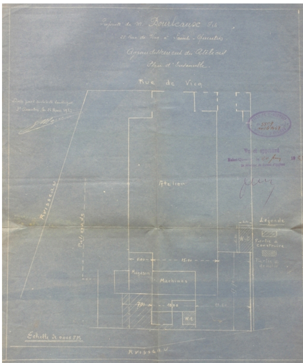
Plan masse de l'usine en 1923 (AC Saint-Quentin).
