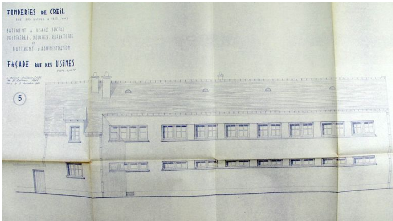
Élévation sur cour de la façade du bâtiment à usage social, par Bailly, 1946 (AD Oise ; 753W28840).
