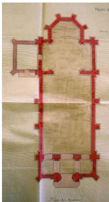
Plan des fondations de la nouvelle église, par Herbault (architecte), 25 avril 1866 (AD Somme ; 99 O 3775). Phot. Fournier Bertrand (reproduction) IVR22_20088015408NUCA
