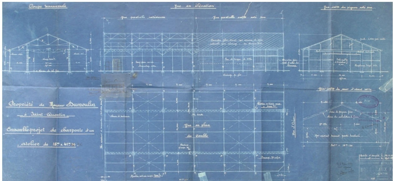
Plan des ateliers projetés, par Bourleaux Fils, 1926 (AC Saint-Quentin).
