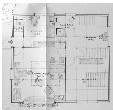
Plan masse du modèle de maison préfabriquée du Groupement Technique du Bâtiment, 1953 (AC Montataire ; 102W4).
