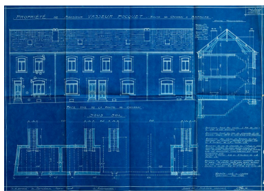
Propriété de M. Vasseur-Poquet, route de Cambrai à Bapaume : face vue de la route de Cambrai, coupe transversale, plan du sous-sol. Signé par Paul Senglet, architecte, M. Vasseur, propriétaire en mai 1926. (AD Pas-de-Calais, 10R9/33, dossier n°476). Phot. Thibaut Pierre (reproduction) IVR32_20216200097NUCA
