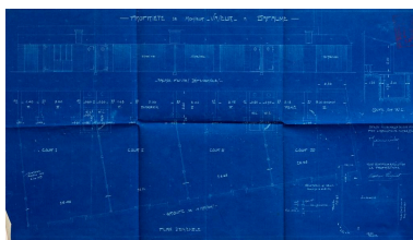
Propriété de M. Vasseur à Bapaume : petites dépendances : façades, plan d'ensemble. Signé et daté par Julien Wirton, architecte, M. Vasseur, propriétaire, le 20 septembre 1929. (AD Pas-de-Calais, 10R9/33, dossier n°476). Phot. Thibaut Pierre (reproduction) IVR32_20216200010NUCA
