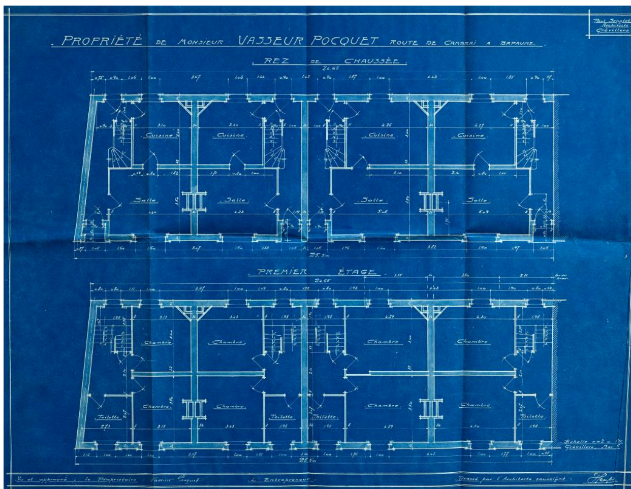
Propriété de M. Vasseur-Poquet, route de Cambrai à Bapaume : plans du rez-de-chaussée et du premier étage. Signé par Paul Senglet, architecte, M. Vasseur, propriétaire en mai 1926. (AD Pas-de-Calais, 10R9/33, dossier n°476).
