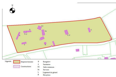
Plan masse et de situation du camping. Dess. Elisabeth Justome IVR22_20058002572NUDA
