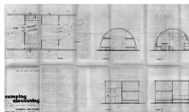
Plans types d'un bungalow (AC Mers-les-Bains). Phot. Thierry Lefébure IVR22_20058000312VB
