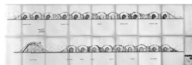
Façades des bungalows et de la salle de réunion, 24 novembre 1972 (AC Mers-les-Bains). Phot. Thierry Lefébure IVR22_20058000314VB
