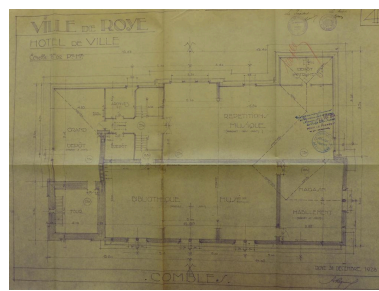
Ville de Roye. Hôtel de ville. Plan des combles. A. Régnier architecte, 1928 (AD Somme ; 99O 3296). Phot. Isabelle Barbedor IVR32_20228005036NUCA
