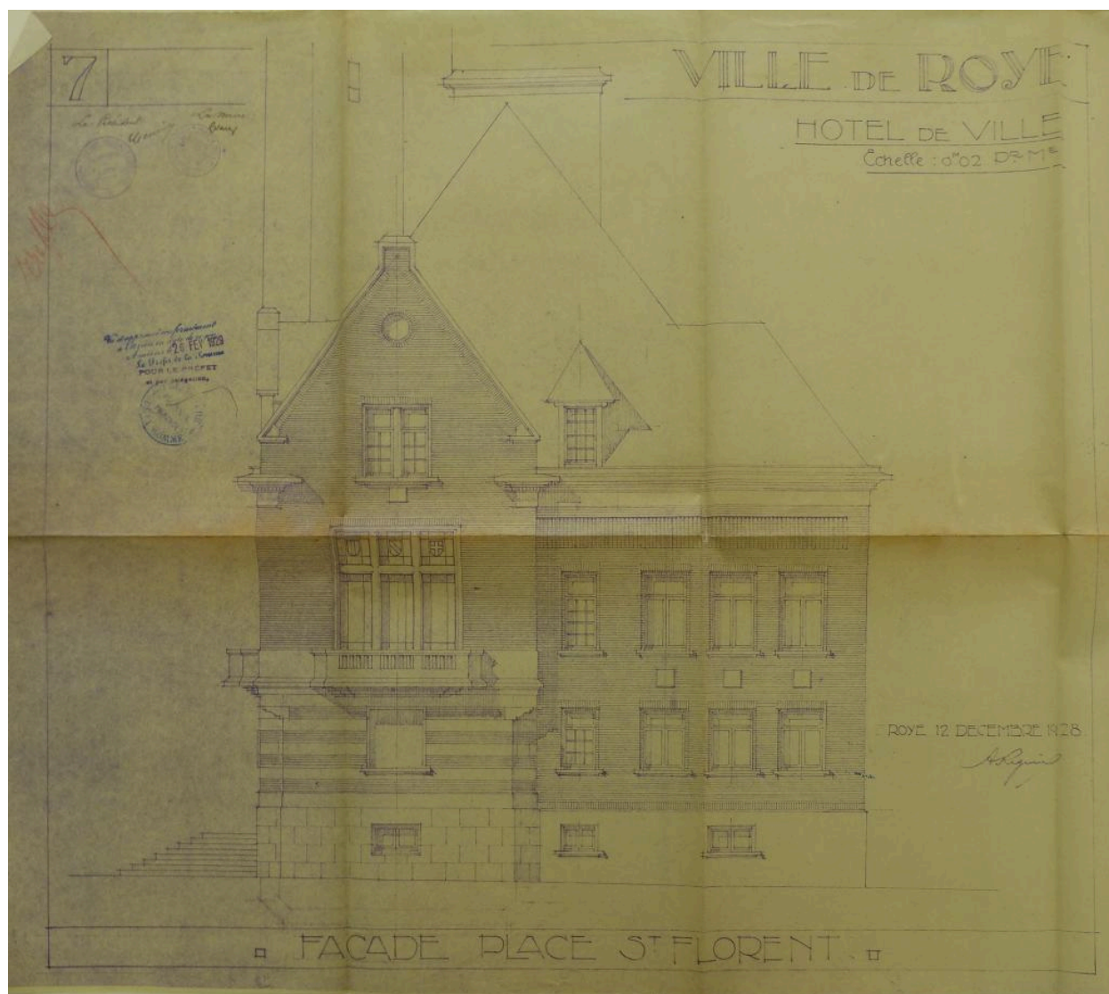
Ville de Roye. Hôtel de ville. Façade place Saint-Florent. A. Régnier architecte, 1928 (AD Somme ; 990 3296).
