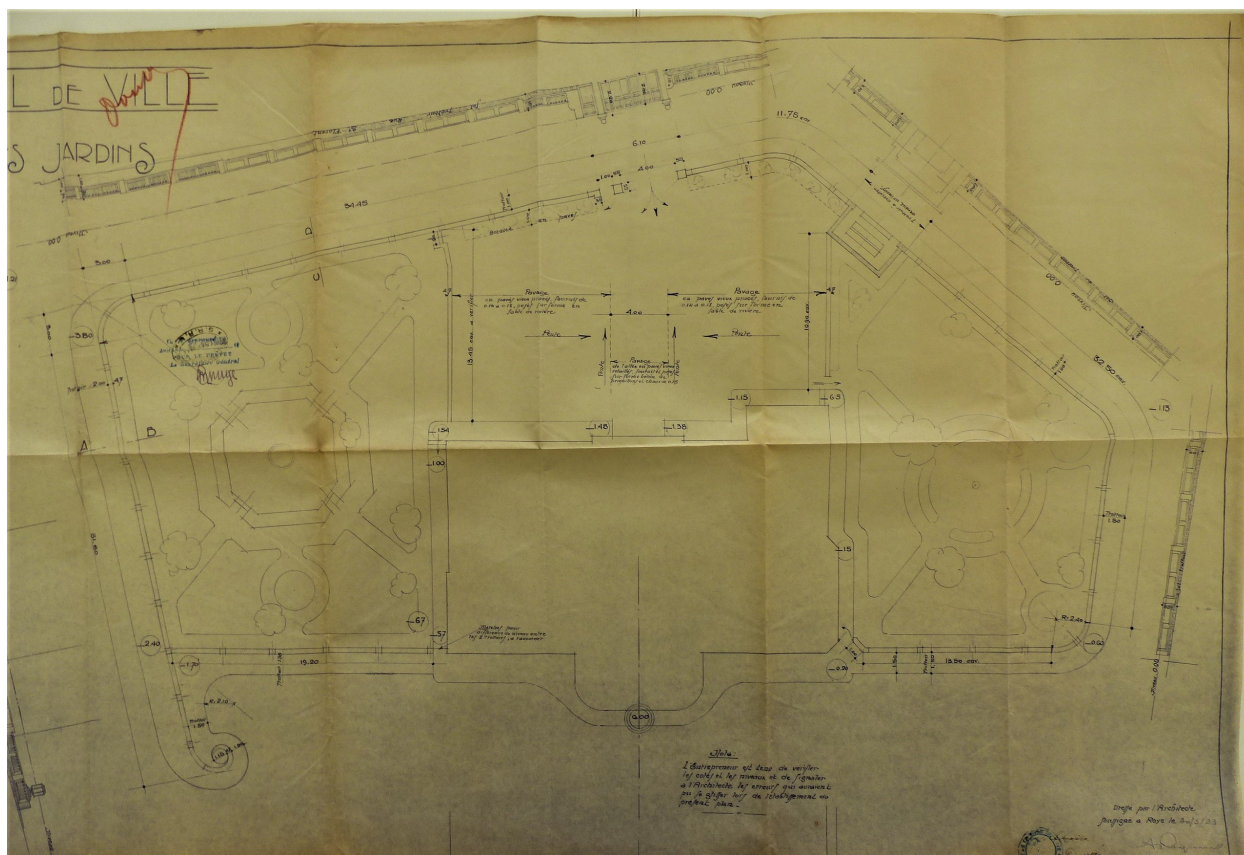
Roye. Hôtel de ville. Entourage des squares. Régnier architecte, 1933 (AD Somme ; 99O 3296).
