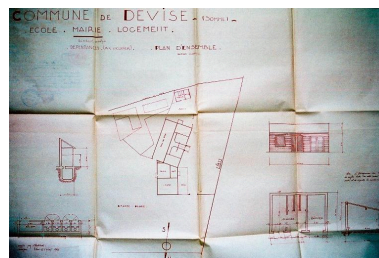
Plan d'ensemble, plan et élévation des dépendances, A. Rischmann (architecte), 1933 (AD Somme ; 99 O 1375). Phot. Gilles-Henri Bailly (reproduction) IVR22_20158005362NUCA
