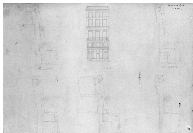
Maison, magasin rue de l'Ecu, actuellement rue Victor Hugo. Plans, coupe, façade signés A. Debayer. B.M. Boulogne- sur-Mer, ms. 535 P, pl. 97. Repro. Philippe Dapvril IVR31_19946200051X
