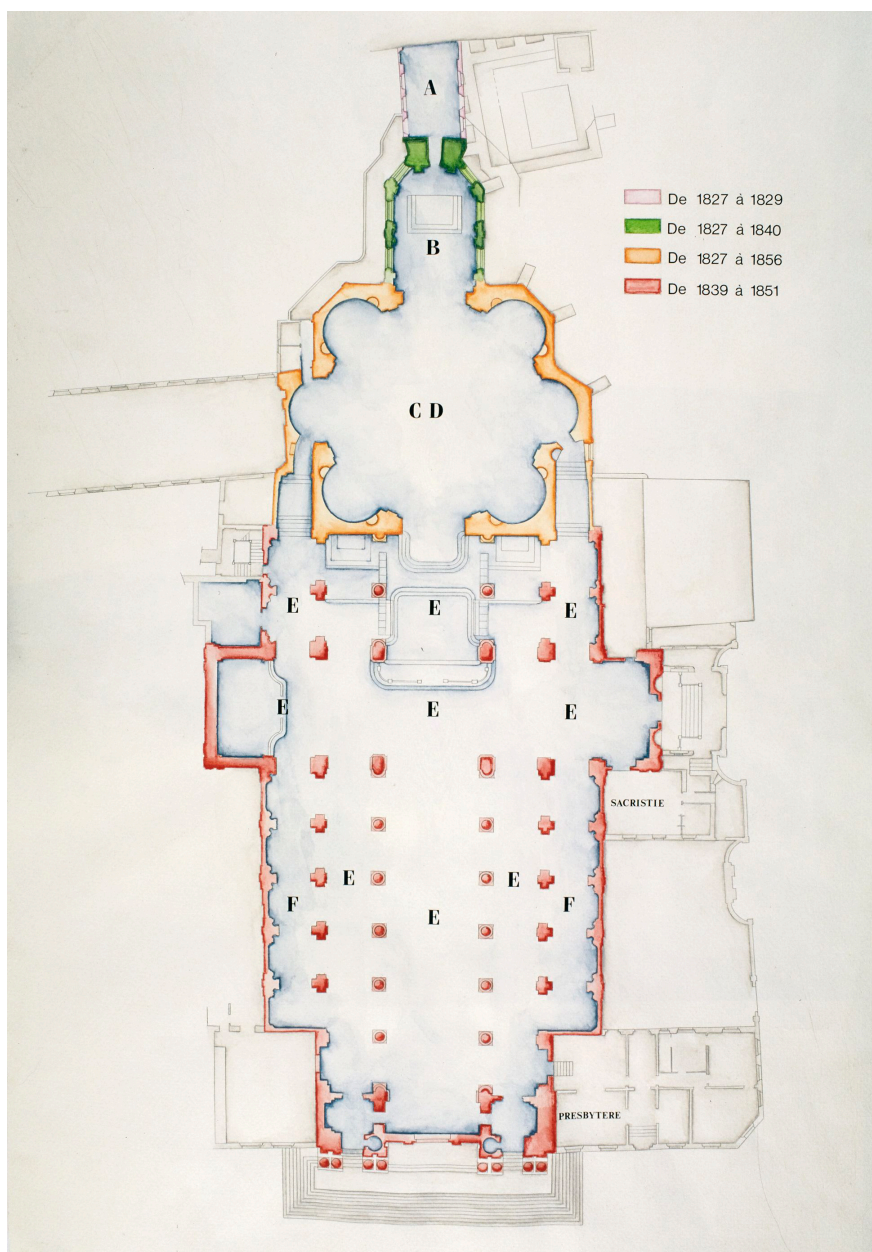
Plan du rez-de-chaussée, plan en couleurs.
