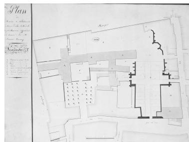
Cathédrale : évêché, plan d'implantation, 1811 (BM Boulogne- sur-Mer, portefeuille 16, n° 8). Repro. Jean-Michel Périn IVR31_19886200475X
