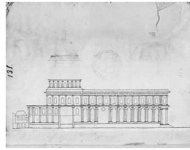
Basilique, étude, façade nord In : Mémoires de Monseigneur Haffreingue, p. 131 (AD Pas-de-Calais ; 9 J 20). Repro. Philippe Caudroit IVR31_19846200029X
