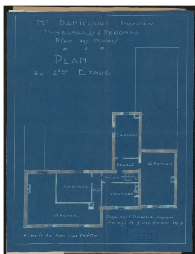
M. Danicourt. Immeuble à Péronne, 1 place des Minimes. Plan du 2e étage, G. Antoine architecte, 1919 (AD Somme ; 10R 1019). Phot. Archives départementales de la Somme IVR32_20228005048NUCA
