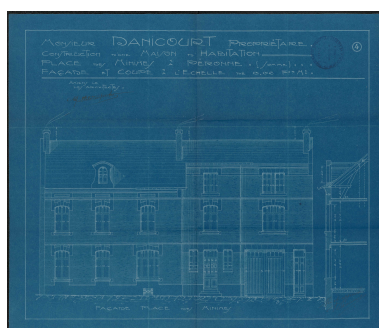
M. Danicourt. Construction d'une maison d'habitation à Péronne, rue des Minimes. Façade et coupe. Mallet et Carpentier architectes (AD Somme ; 10R 1019). Phot. Archives départementales de la Somme IVR32_20228005045NUCA
