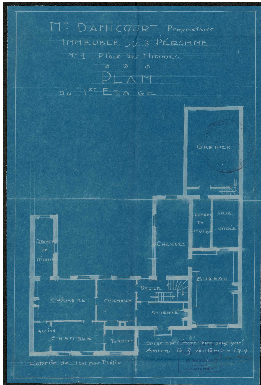
M. Danicourt. Immeuble à Péronne, 1 place des Minimes. Plan du 1er étage, G. Antoine architecte, 1919 (AD Somme ; 10R 1019).
