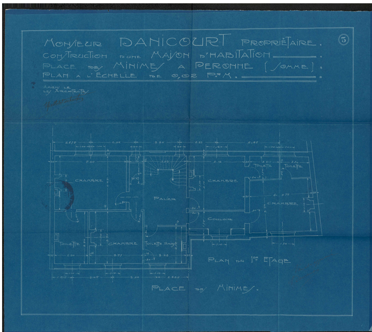
M. Danicourt. Construction d'une maison d'habitation à Péronne, rue des Minimes. Plan du 1er étage. Mallet et Carpentier architectes (AD Somme ; 10R 1019).
