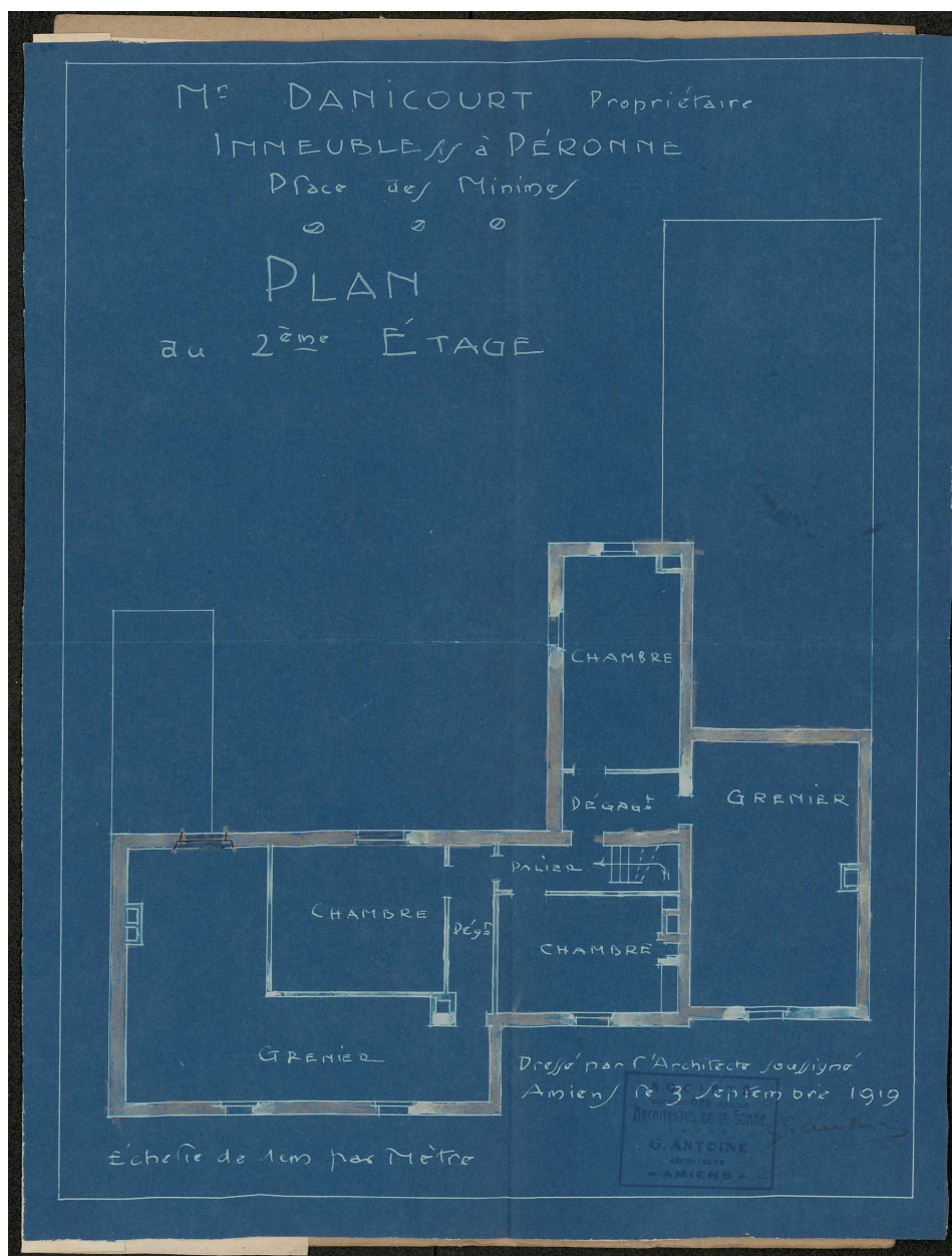
M. Danicourt. Immeuble à Péronne, 1 place des Minimes. Plan du 2e étage, G. Antoine architecte, 1919 (AD Somme ; 10R 1019).
