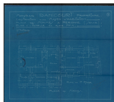
M. Danicourt. Construction d'une maison d'habitation à Péronne, rue des Minimes. Plan du 1er étage. Mallet et Carpentier architectes (AD Somme ; 10R 1019). Phot. Archives départementales de la Somme IVR32_20228005043NUCA
