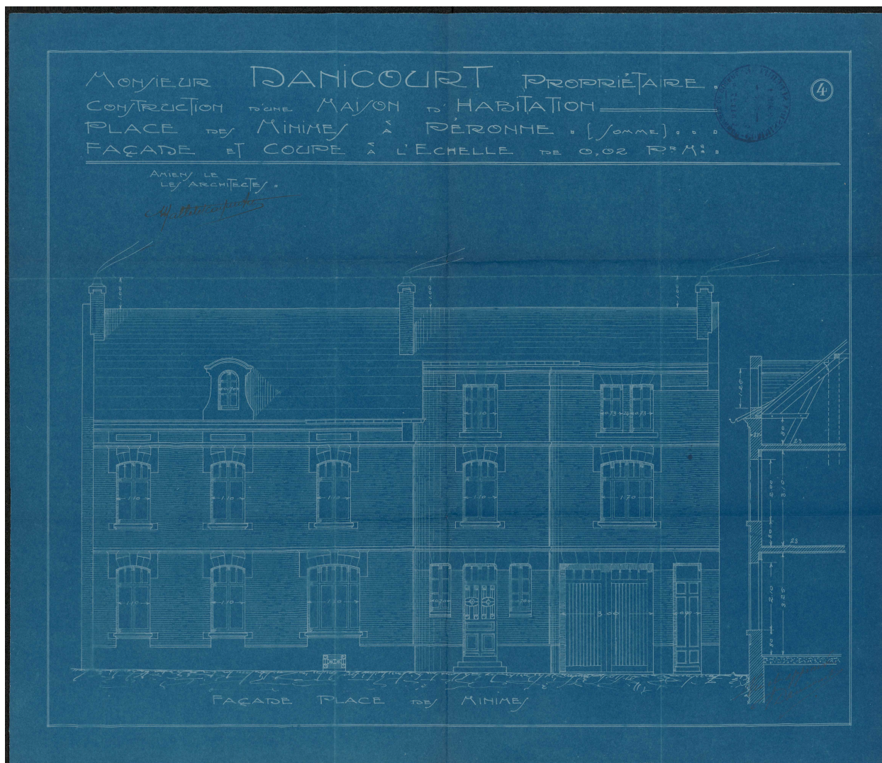
M. Danicourt. Construction d'une maison d'habitation à Péronne, rue des Minimes. Façade et coupe. Mallet et Carpentier architectes (AD Somme ; 10R 1019).
