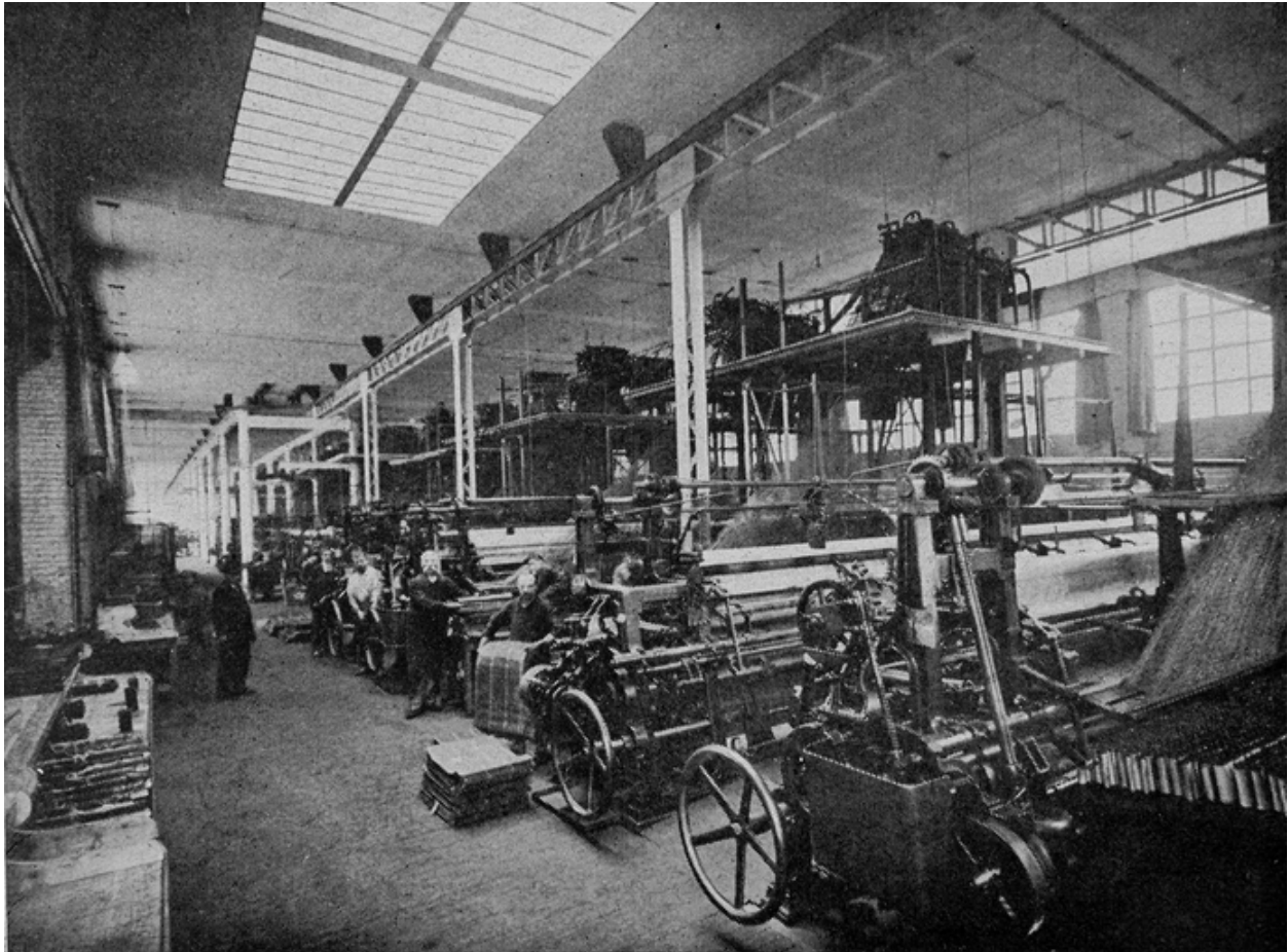
Intérieur des ateliers reconstruits (vers 1920-1921) : alignement de métiers à guipure (Le Monde Illustré).
