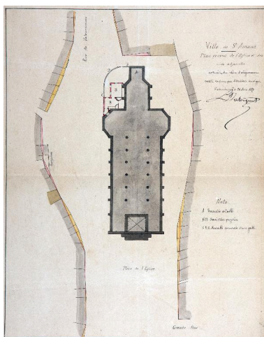
Le plan de l'église et sa situation avec les rues adjacentes, Louis Dutouquet architecte, 1870 (AD Nord Série 2 O 525/94). Phot. Pierre Thibaut IVR31_20135900076NUCA
