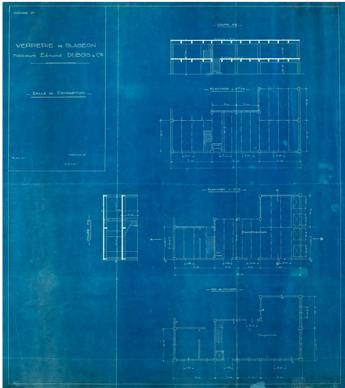
Verrerie de Glageon de MM Edmond Dubois et Cie. Salle de composition. Plan de coupes et planchers, non daté (circa 1920).
