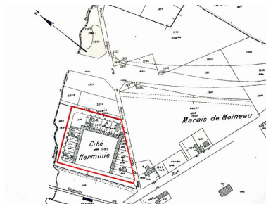
Plan d'ensemble, extrait du plan cadastral de la commune, section C, 4e feuille, 1/1250e.
