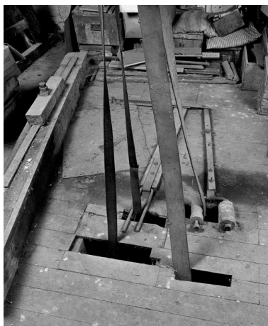
Courroies de transmission, en comble. Phot. Olivier Coquelle IVR22_19946000903X
