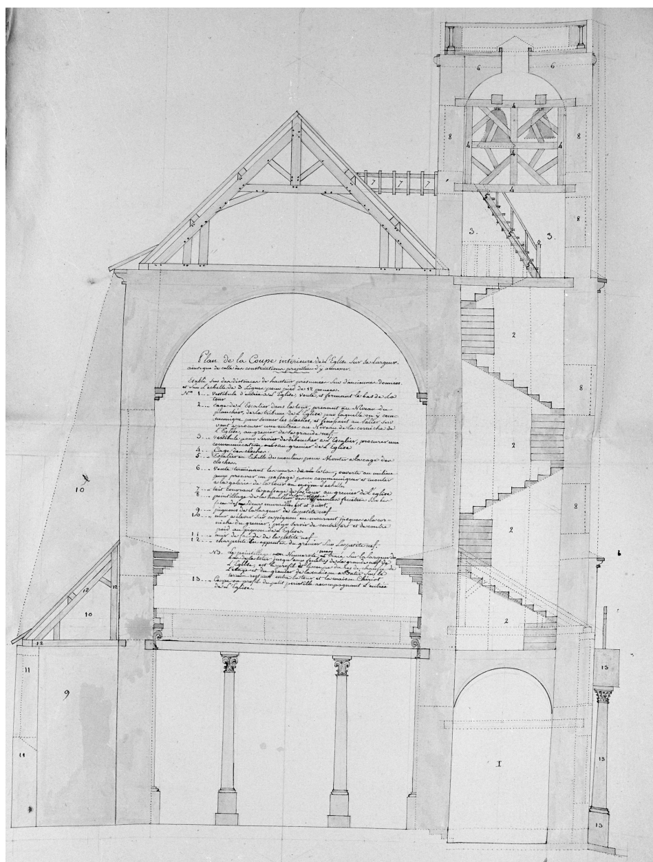
Eglise, clocher, coupe transversale (A.D. Pas-de-Calais, 9 J 2 OP 91, pl. 3).
