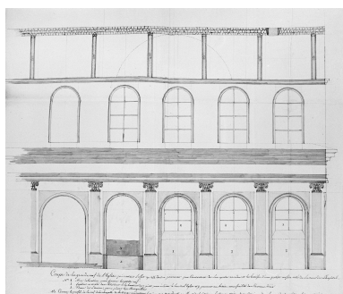
Eglise, coupe longitudinale partielle, projet vers 1810 (A.D. Pas-de-Calais, 9 J 2 OP 91). Phot. Jean-Michel Périn IVR31_19886200555X
