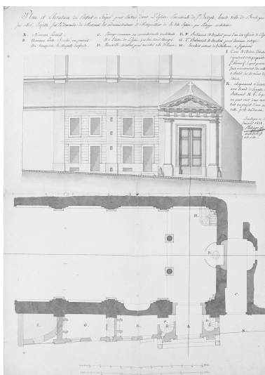
Eglise, croquis, projet daté 1808 (A.D. Pas-de-Calais, 9 J 2 OP 91). Phot. Jean-Michel Périn IVR31_19886200554X
