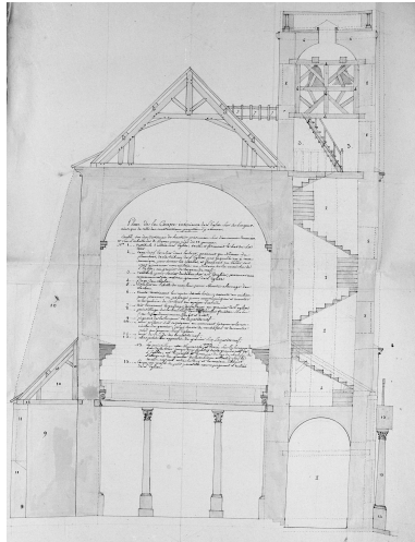
Eglise, clocher, coupe transversale (A.D. Pas-de- Calais, 9 J 2 OP 91, pl. 3). Phot. Jean-Michel Périn IVR31_19886200523X
