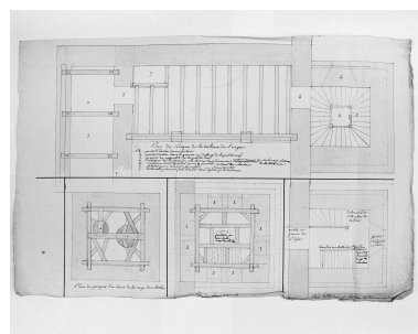
Eglise, clocher, projet, plans des niveaux, dessinés par M. Depestre (A.D. Pas-de-Calais, 9 J 2 OP 91, pl. 2). Phot. Jean-Michel Périn IVR31_19886200524X
