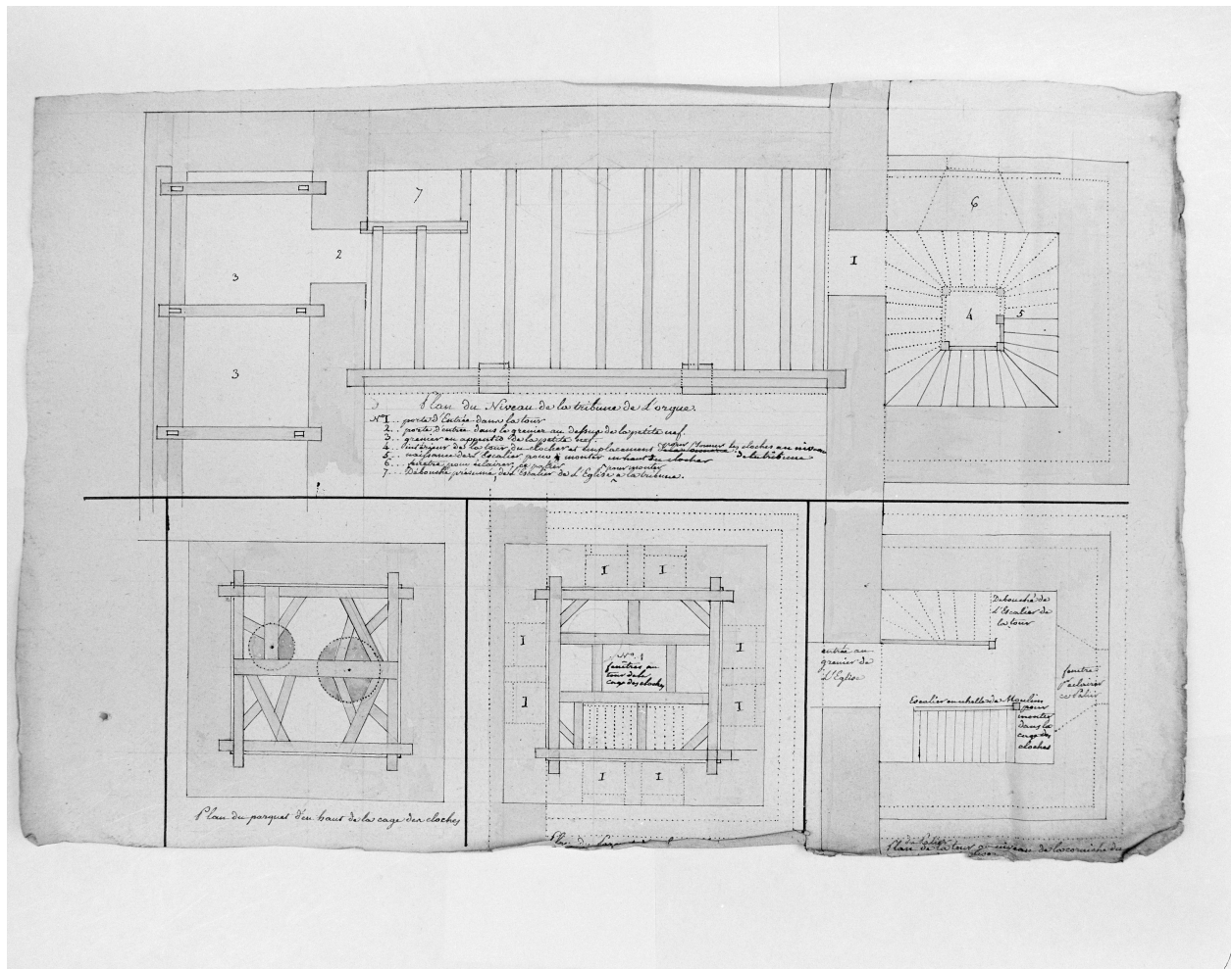
Eglise, clocher, projet, plans des niveaux, dessinés par M. Depestre (A.D. Pas-de-Calais, 9 J 2 OP 91, pl. 2).
