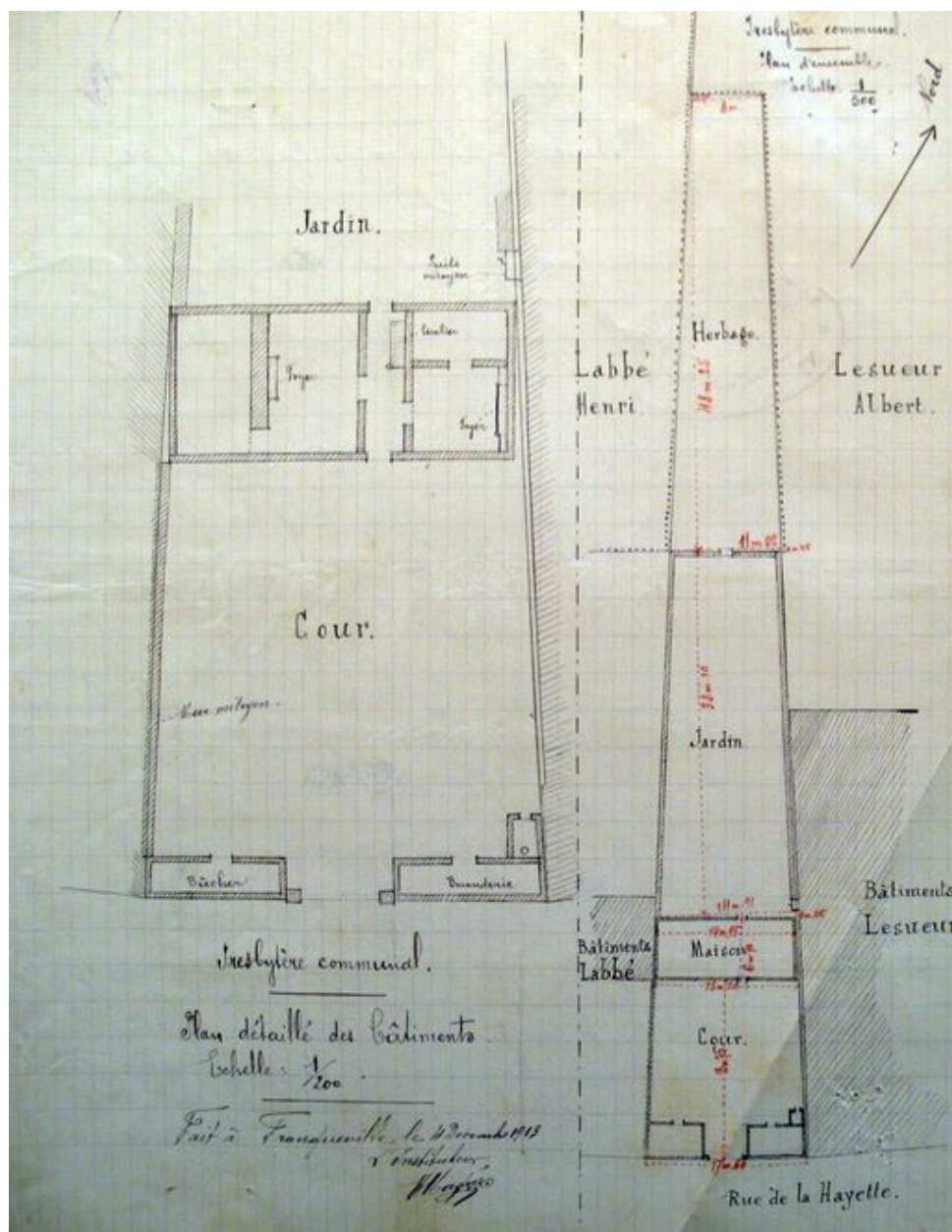
Plan de la parcelle et plan au sol du presbytère, par Magner, 1913 (A.D Somme ; 99 O 1817).
