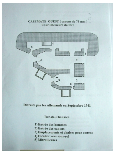
Plan de la casemate ouest (Archivées Privées). Phot. Sophie Luchier IVR31_20045905446NUC
