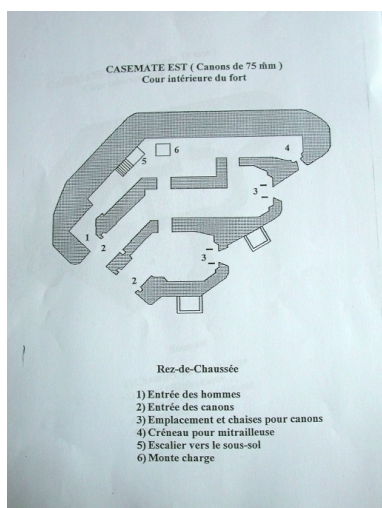
Plan de la casemate est (Archivées Privées). Phot. Sophie Luchier IVR31_20045905445NUCA
