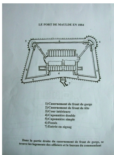
Plan du fort en 1884 (Archivées Privées). Phot. Sophie Luchier IVR31_20045905443NUC
