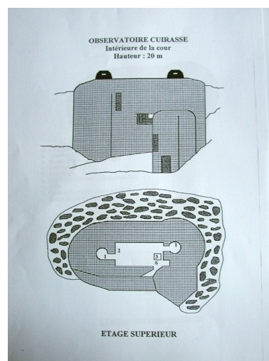
Plan de l'observatoire cuirassé (Archivées Privées). Phot. Sophie Luchier IVR31_20045905447NUC
